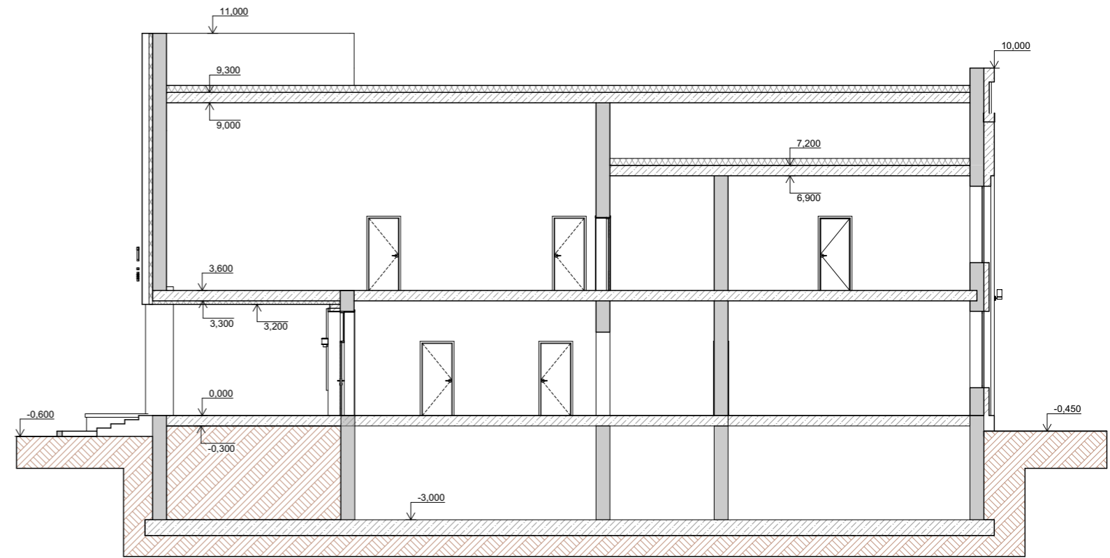
Разрез 2-2
